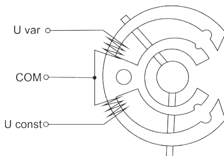
Рисунок 11. Индуктивные датчики положения рейки
