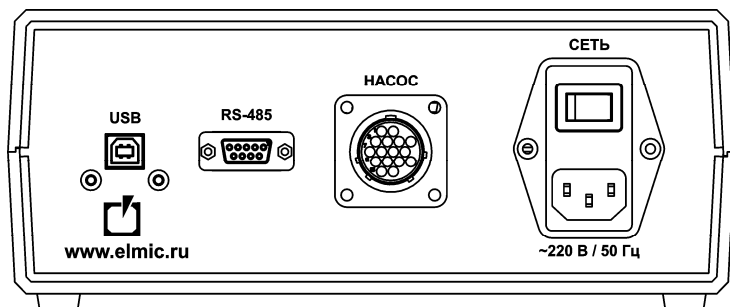
Рисунок 2. Панель задняя
