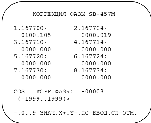
Рисунок 4.33 - Настройка коррекции фазы выбранного канала SB-457M
