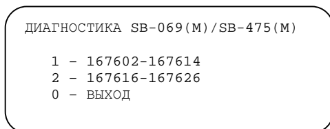
Рисунок 4.25 -Выбор диапазона адресов внешних плат дискретных входов
