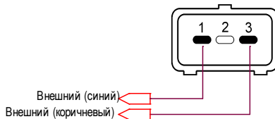
Рисунок 15. Схема распайки разъема ТНВД тип 3
