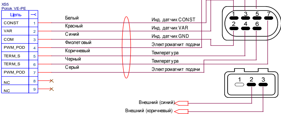
Рисунок 11. Схема распайки разъема ТНВД тип 1
