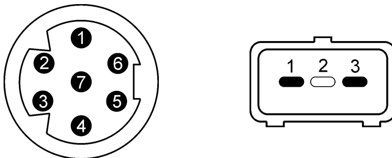
Рисунок 14. Разъем ТНВД тип 3: а – подача и индуктивный датчик, б – клапан опережения
